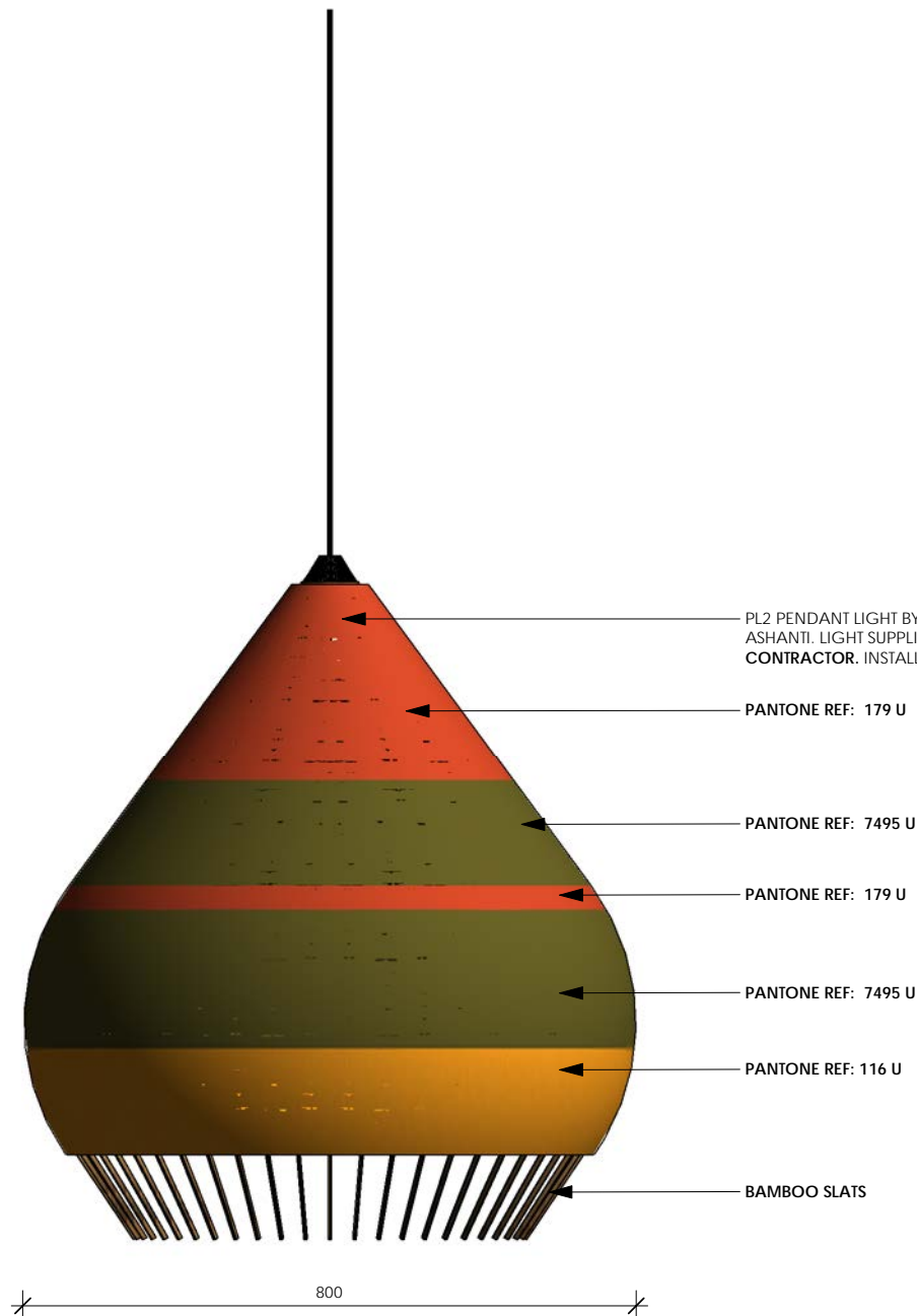
2 PL2 PENDANT ELEVATION 220 1 : 10
